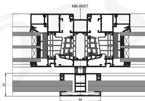
srednji okenski profil, pogled
