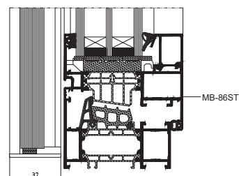
okno z ograjo tipa H, pogled od spodaj
