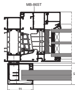
okno z ograjo, stranski pogled
